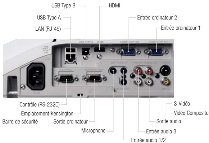
Entrée audio 1/2
